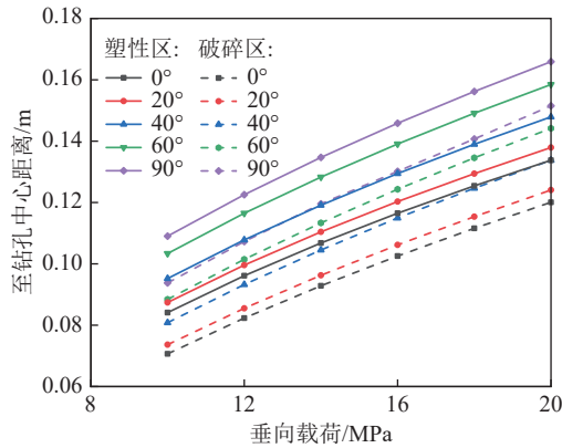
图6 塑性区、破碎区半径随垂向载荷变化曲线
