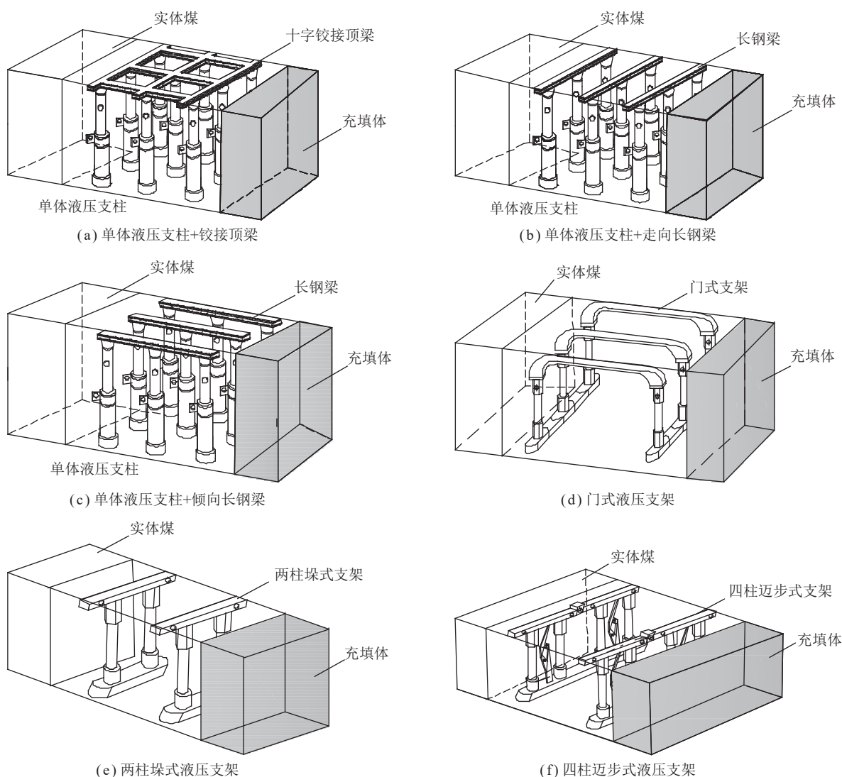
图 4 沿空留巷巷内加强支护类型
