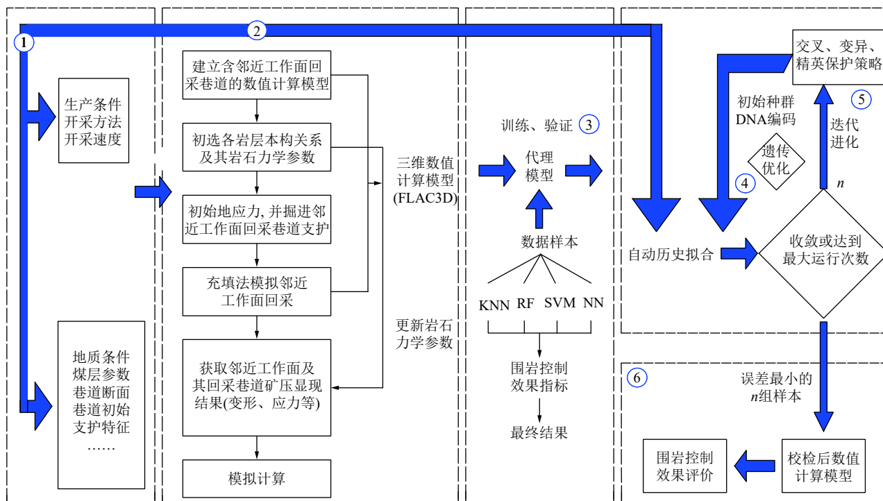
图 9 沿空留巷数值模拟岩石力学参数智能反演工作流
