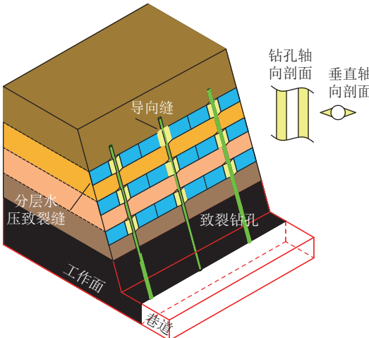
(b) 沿高度方向定向分组致裂
