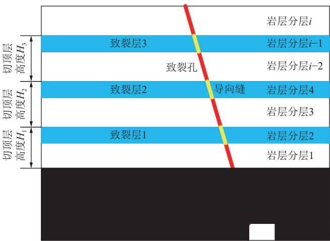
(a) 沿空留巷分组有控切顶
