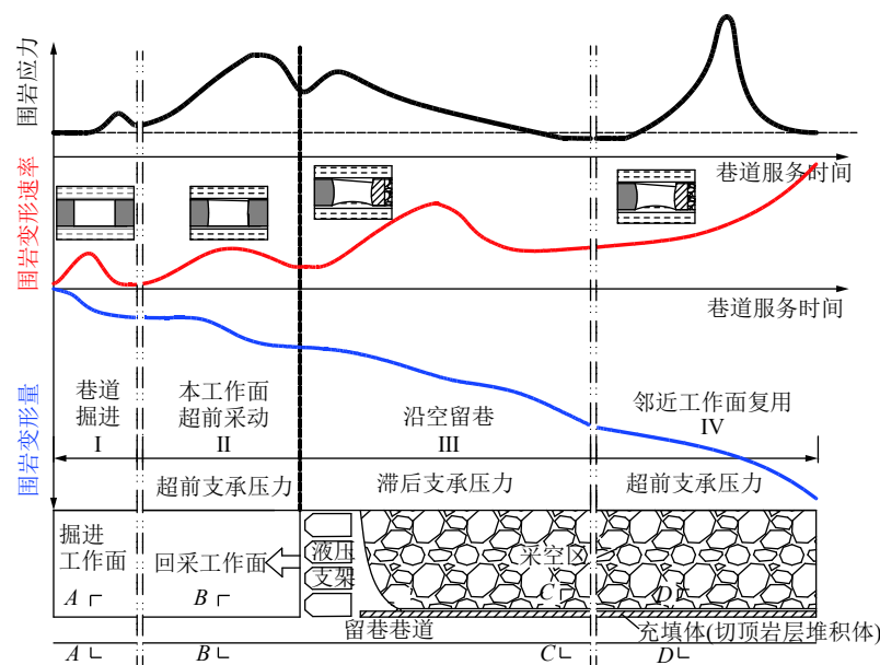
图 2 沿空留巷全周期内围岩变形量、变形速率和应力演化规律
