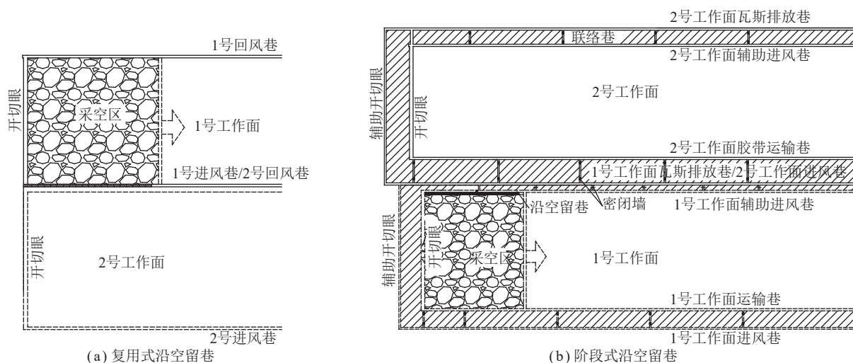
图 1 典型沿空留巷类型
