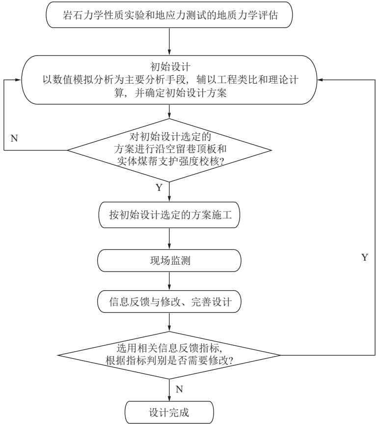
图 3 沿空留巷巷内锚杆支护设计流程
