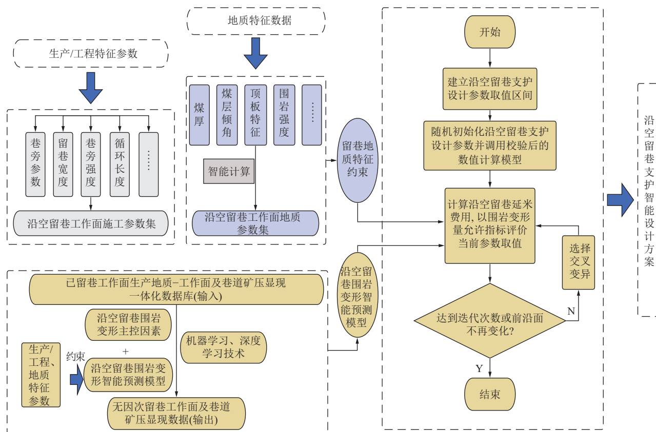
图 10 沿空留巷支护参数智能优选设计思路
