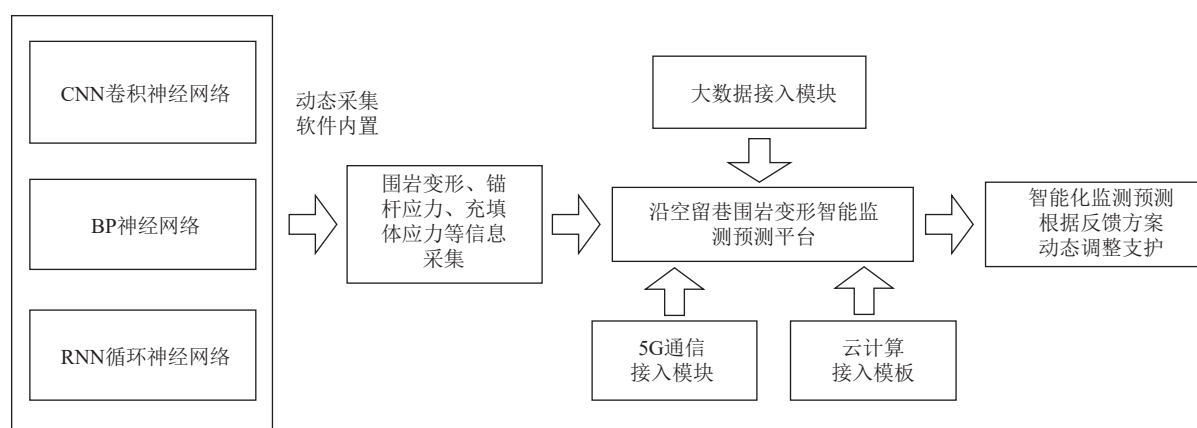
图 8 厚煤层综放/一次采全高沿空留巷有控切顶-充填围岩协同控制示意
